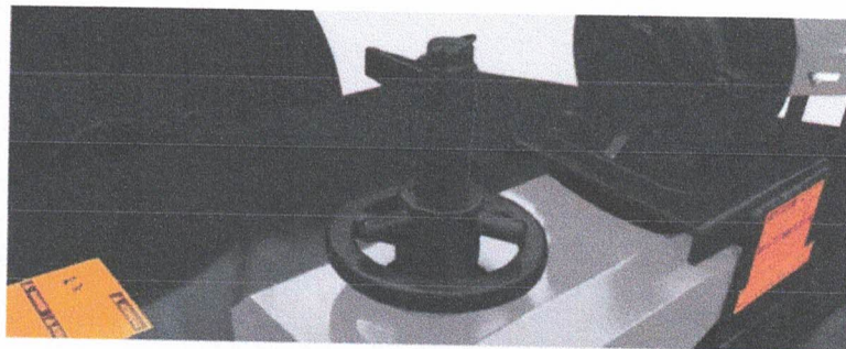
Sistema de regulação das facas através de mandril, que regula altura de corte de 100mm a 320mm. Blade adjustment by thread axle that provide adjustment from 100mm to 320mm. Soporte para la regulación de la altura de corte de las cuchillas, desde 100 hasta 320mm.
