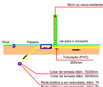
Esquema de Ramal e Alimentador Predial Sílica
