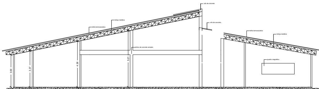
Corte transversal ab Esc: 1:75
